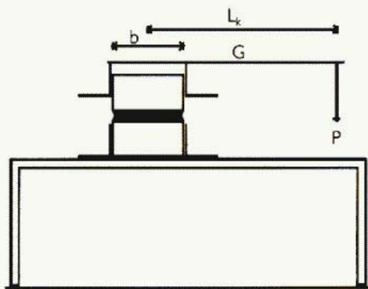
Figur 1. Principskitse for apparatur
